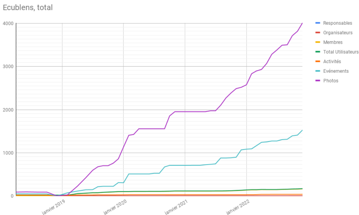
Progression de l'utilisation de resoli.ch depuis janvier 2019
