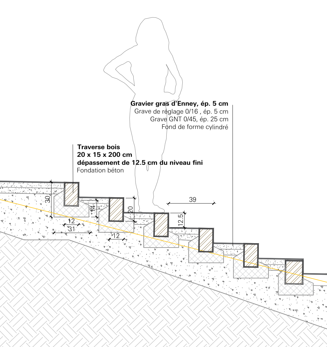
Détail escalier - 1/120
