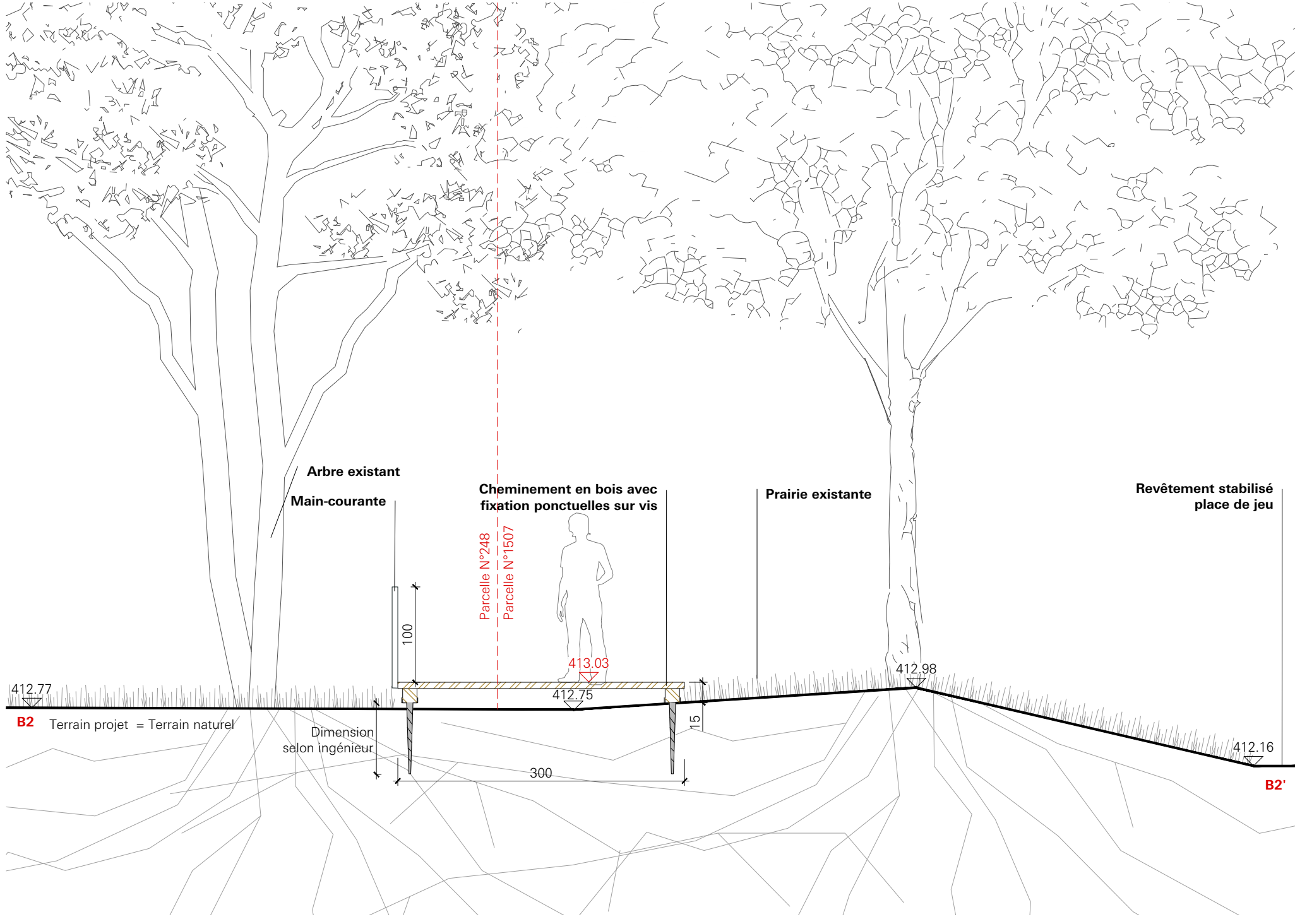
Coupe B2-B2' - 1/50
