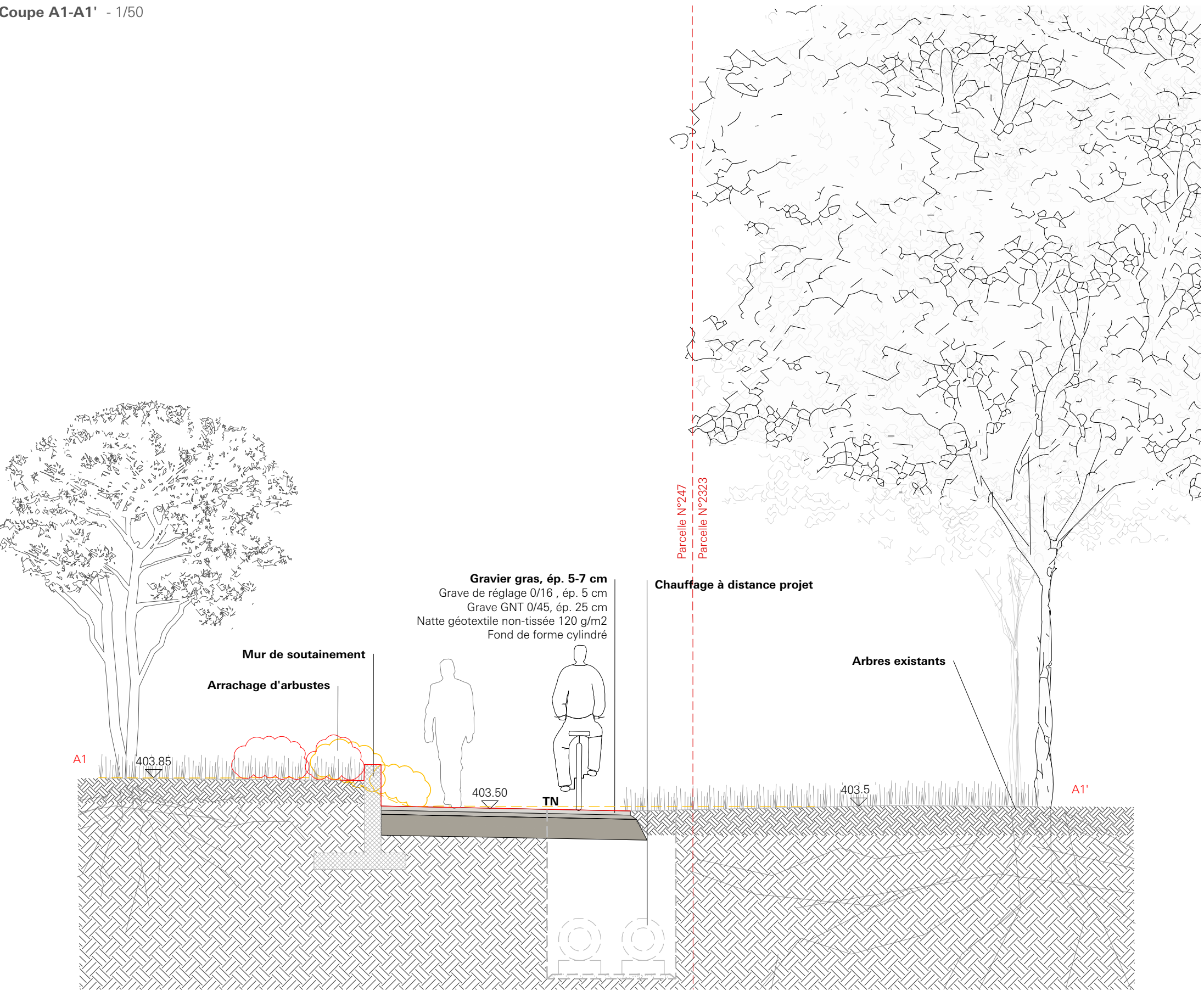
Coupe A1-A1' - 1/50
