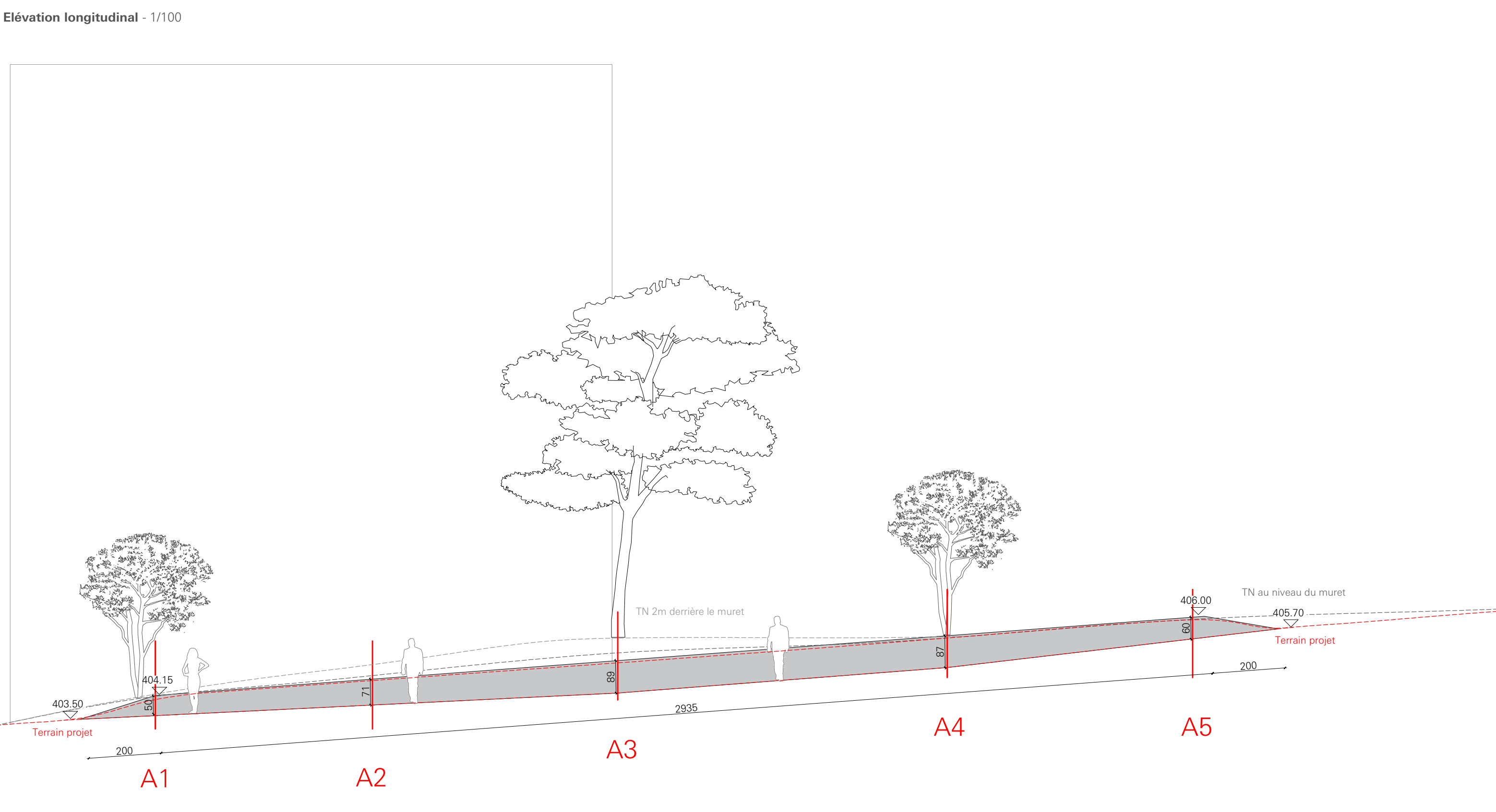
Élévation longitudinale - 1/100
