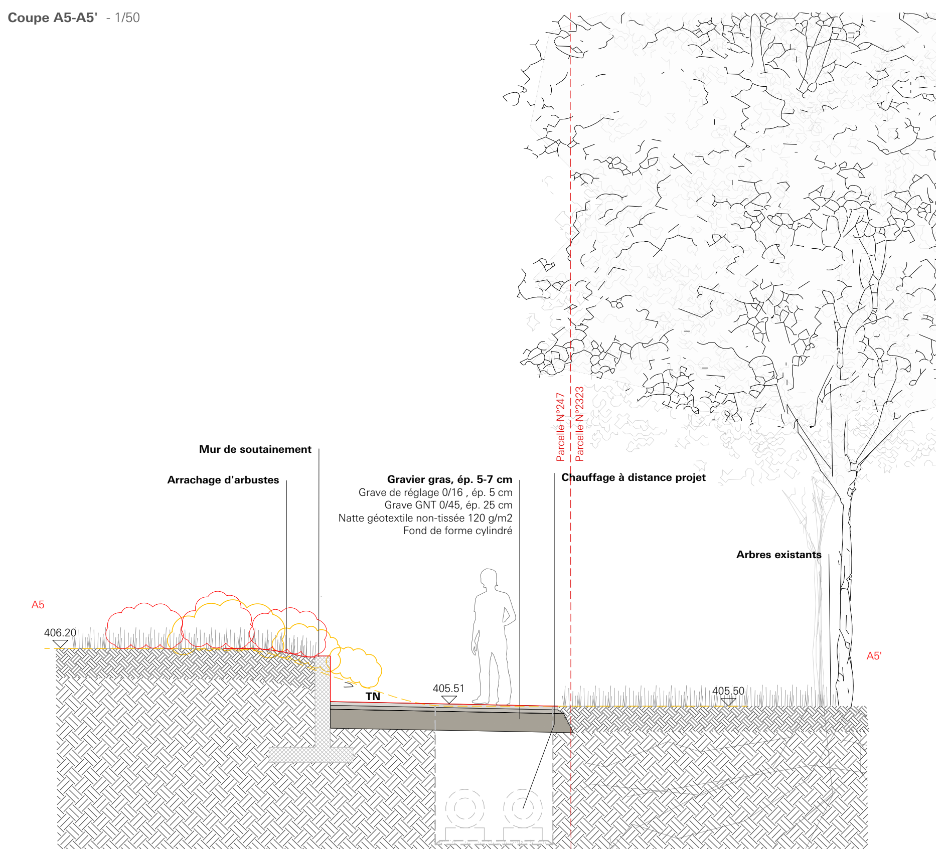
Coupe A5-A5' - 1/50
