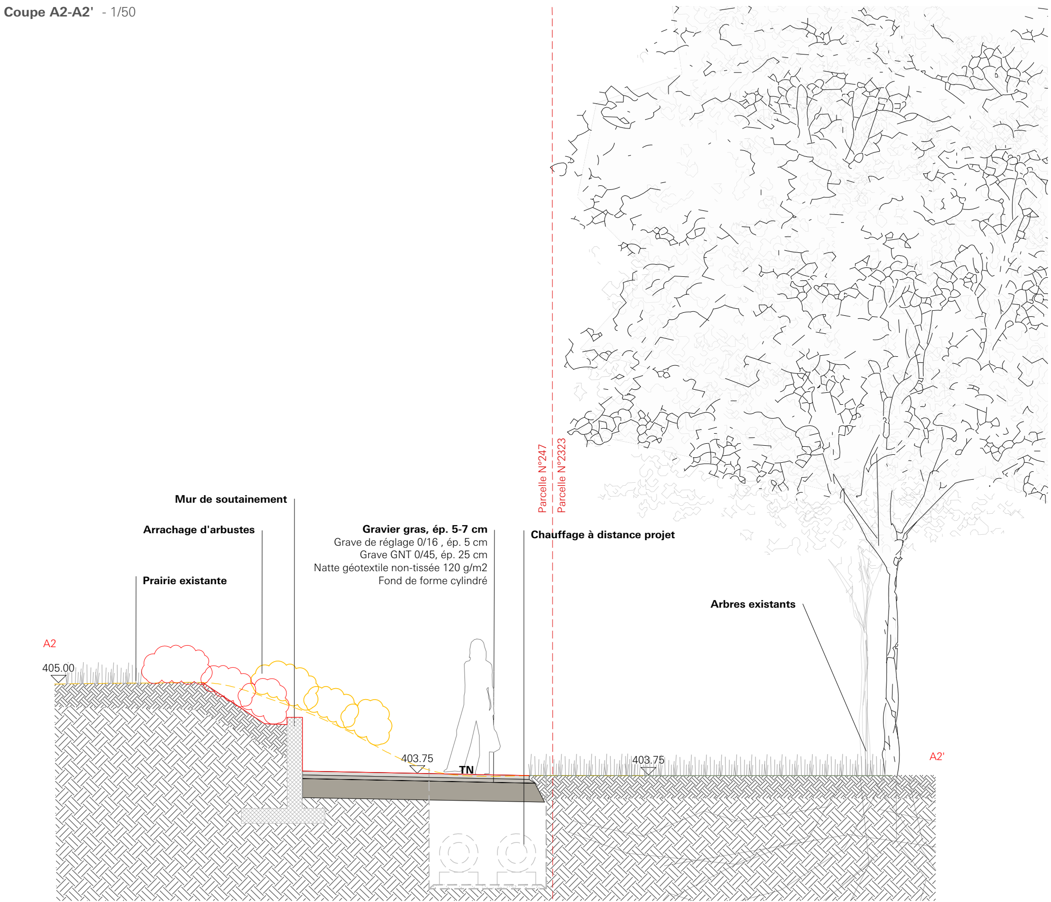
Coupe A2-A2' - 1/50
