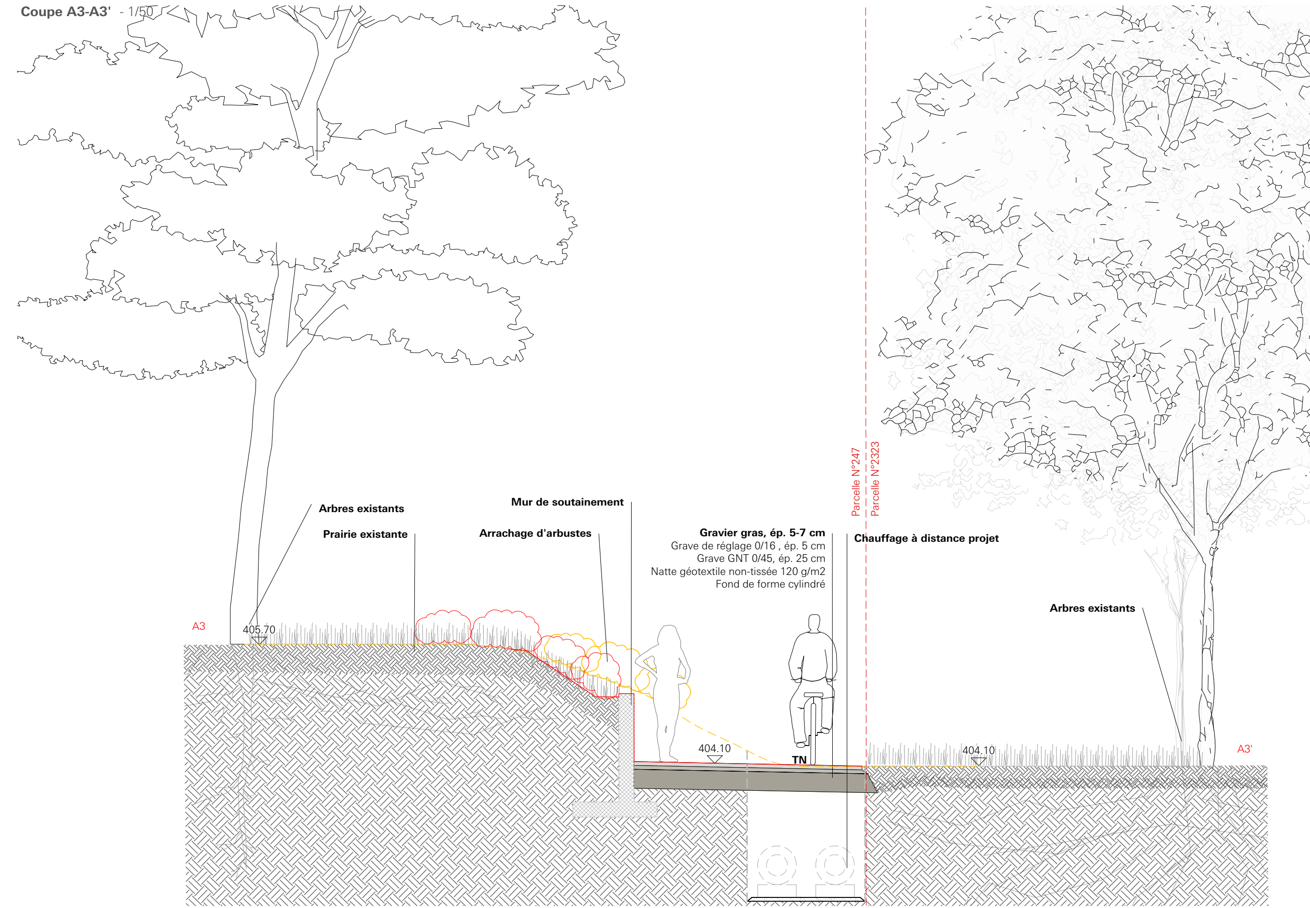
Coupe A3-A3' - 1/50
